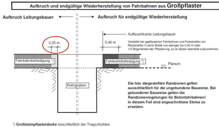
Anlage 4 §7 Berliner Straßengesetz Großpflaster, bei Kleinpflaster 0,15 statt 0,20 m
