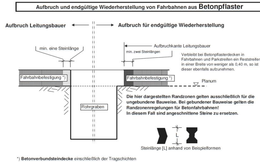
Anlage 6 §7 Berliner Straßengesetz Betonpflaster
